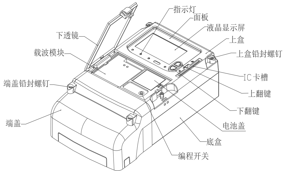
图 2：外形布局图
