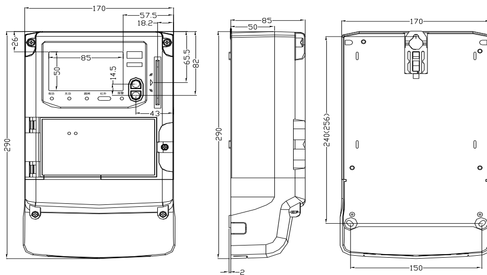
图 3：安装尺寸图
