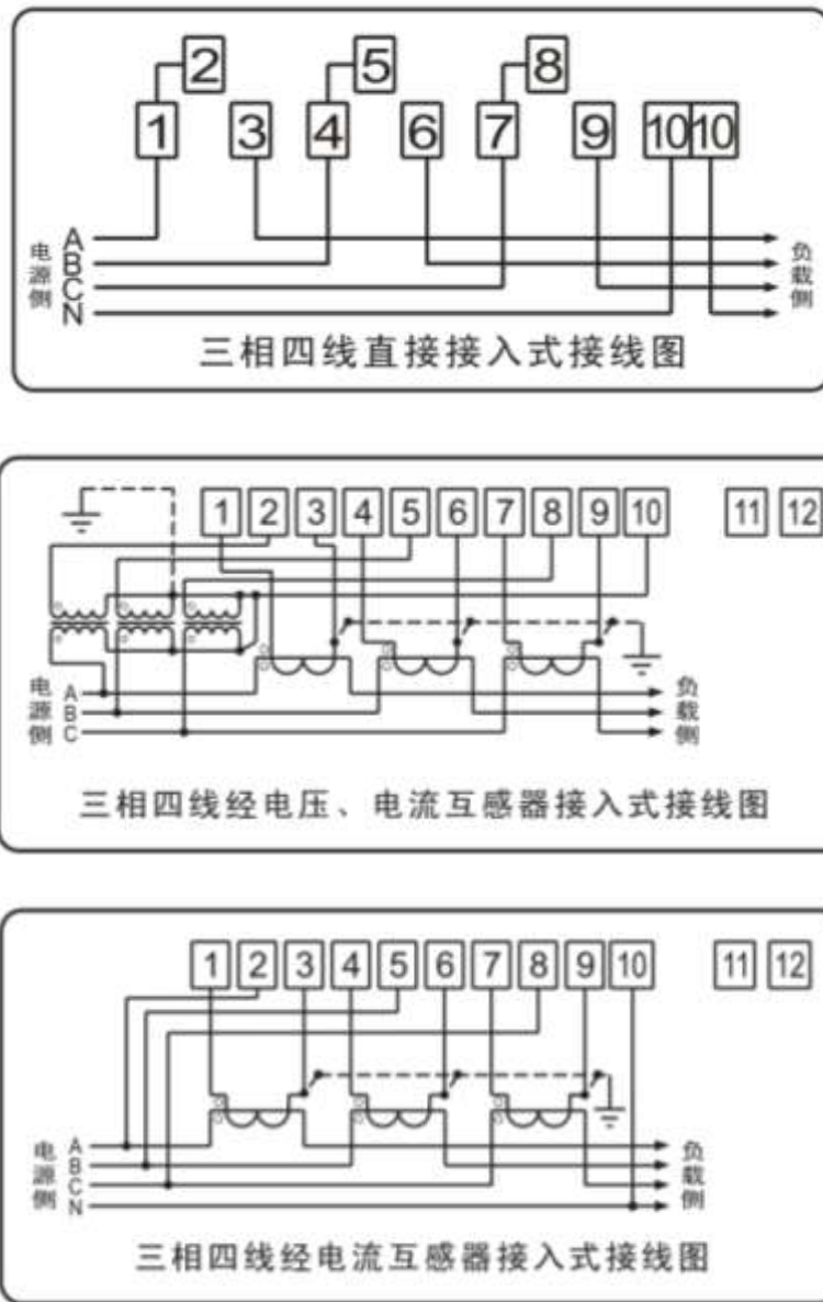
图 4：接线图
