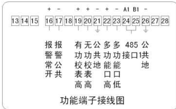
图 7C: 内继电器电能表单 485 辅助端子排列图
