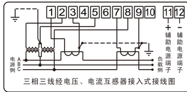
图 4：接线图
