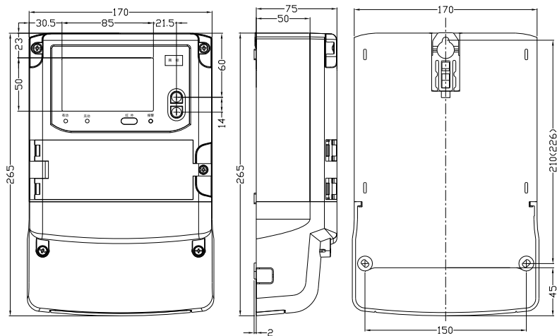
图 3：安装尺寸图
