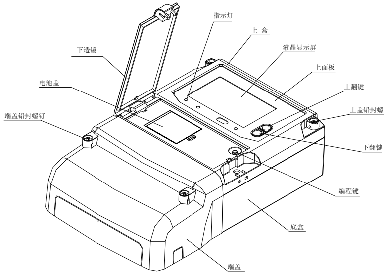
图 2：外形布局图
